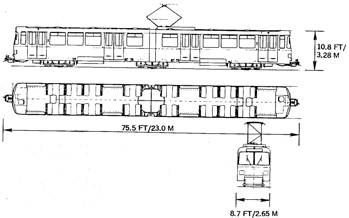
Figure 27. DuWag U2
