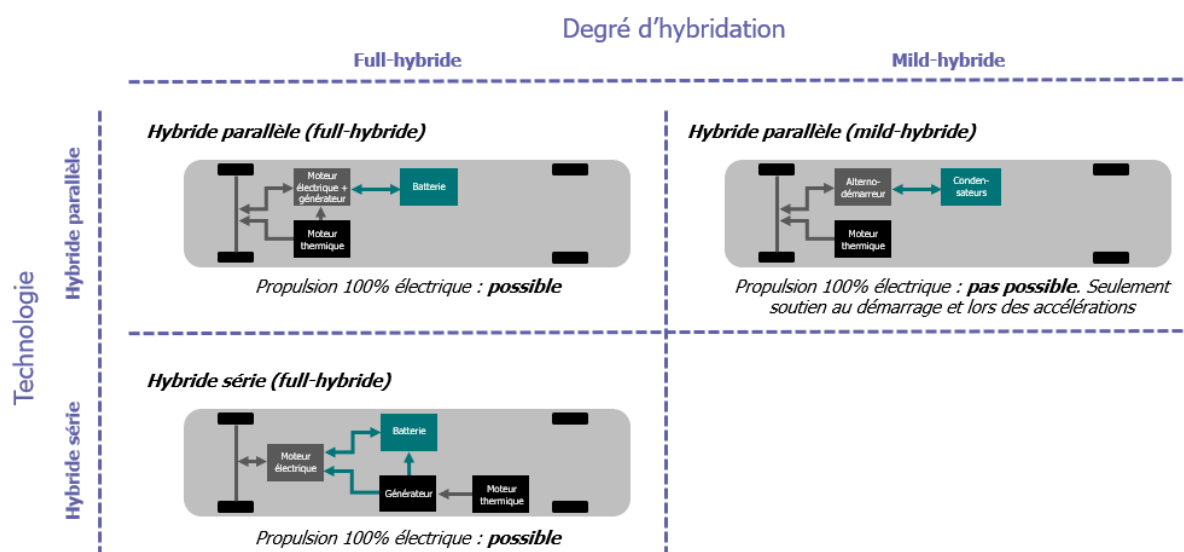
Fig : Technologies de véhicules hybrides
