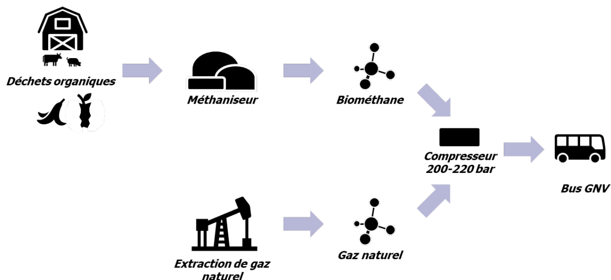
Fig : Principe de base du GNV
