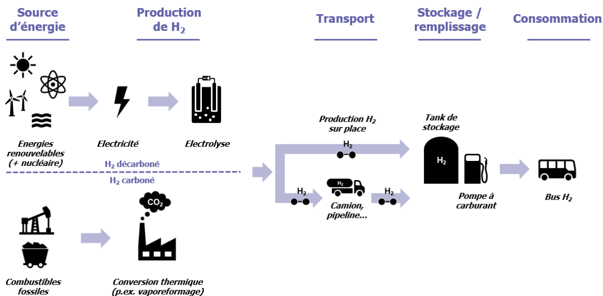
Fig : Chaîne de production de l'hydrogène
