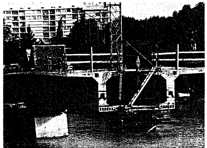
Fig. 9. En attendant la deuxième ligne de tramway, les travaux de l'axe lourd centre-sud se poursuivent : lancement du nouveau pont de Pirmil, automne 1985 (photo SÉMITAN).
