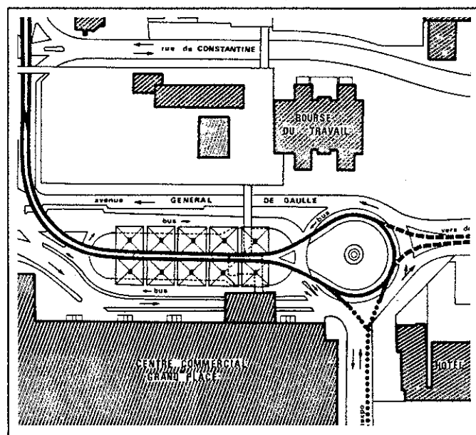
Fig. 6 et 7. Plan du terminus de Grand'Place, à la Villeneuve (document Méttram) et vue des travaux de construction de la boucle de retournement (Photo B. Gournay).
