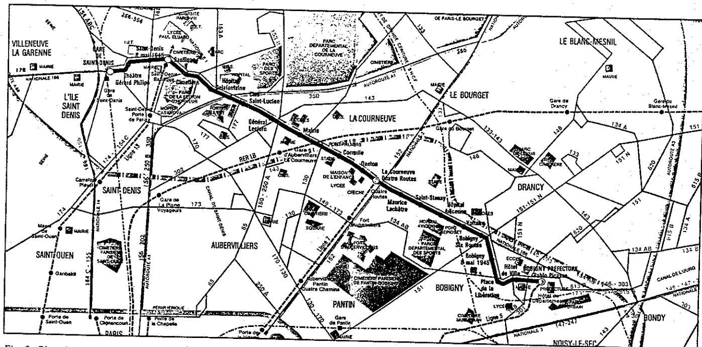
Fig. 2. Plan de situation de la ligne de tramway. Celle-ci sera en correspondance étroite en quatre points avec le réseau ferré de la capitale : terminus des lignes 5, 7 et 13 du métro, gare SNCF de St-Denis (document RATP).
