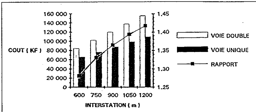
Figure 10. Coût d'interstation en cadre superficiel pour le matériel M3.
