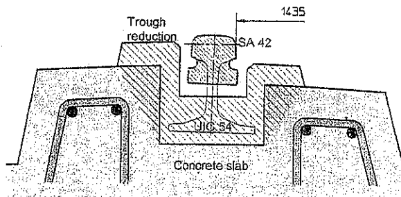
Fig. 6: Low nose SA 42
