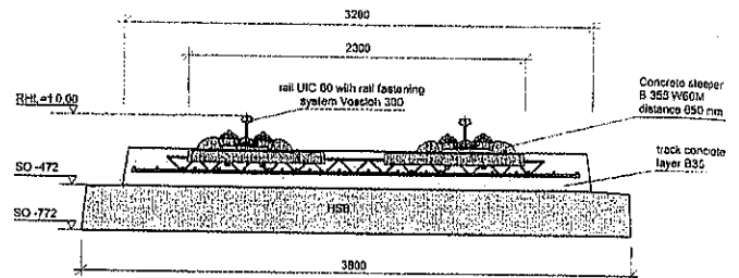
Fig. 2: Rheda 2000
